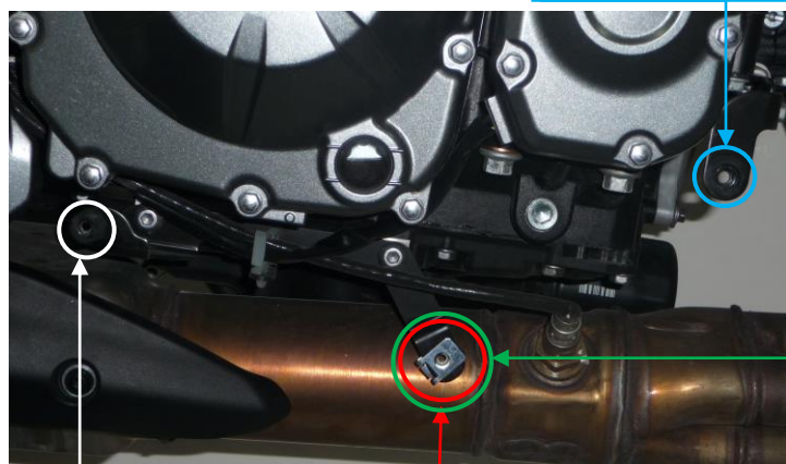
Position de la vis 5×20
