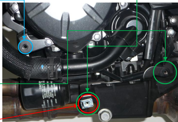
Position des entretoises plastique
